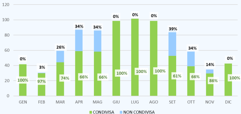
Figura 4: energia mensile della configurazione
